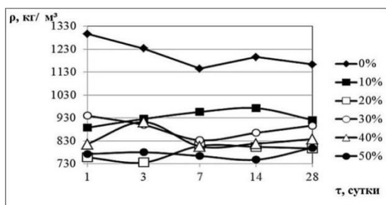
Рис. 6 График зависимости плотности образцов, с добавкой шлама, обожжённого при 900 °С, от количества добавки
