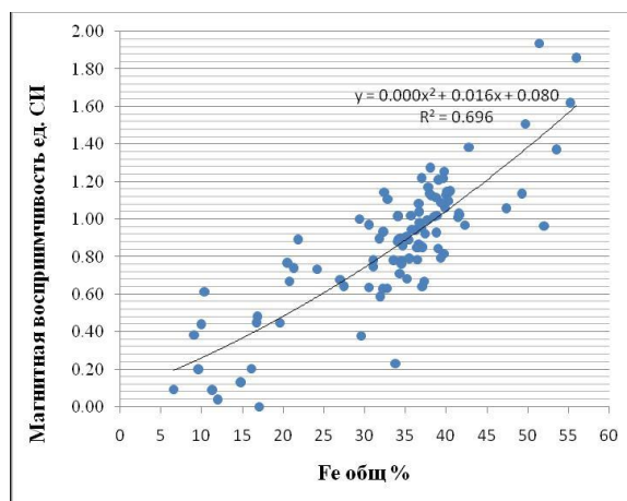
Рис. Зависимость магнитной восприимчивости от общего содержания железа в железистых кварцитах Верхнеомолонского месторождения
