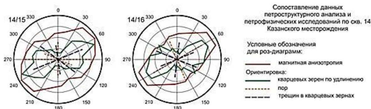
Рис. 2. Сопоставление данных петроструктурного анализа и петрофизических исследований по скважине 14 Казанского месторождения
