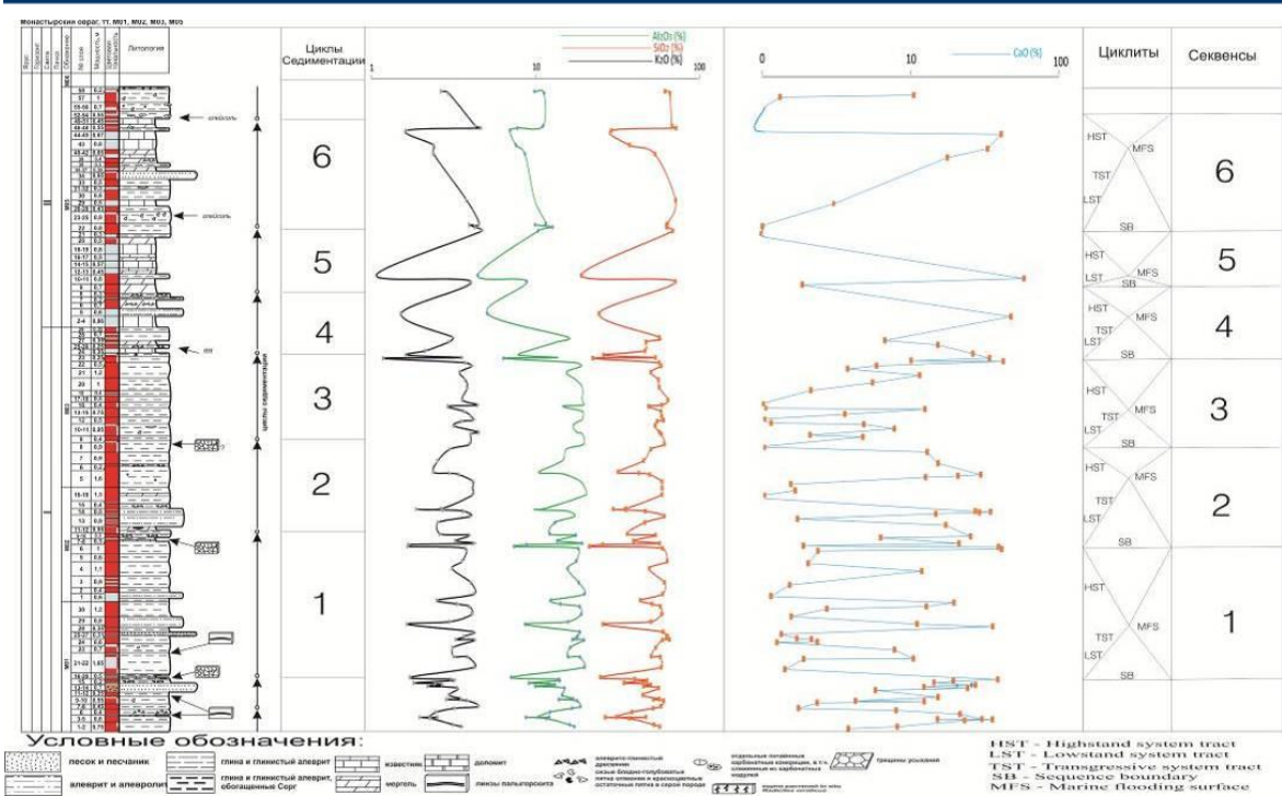
Рис. 3 Разрез первой и второй свиты Уржумского яруса в овраг.Монастырский
