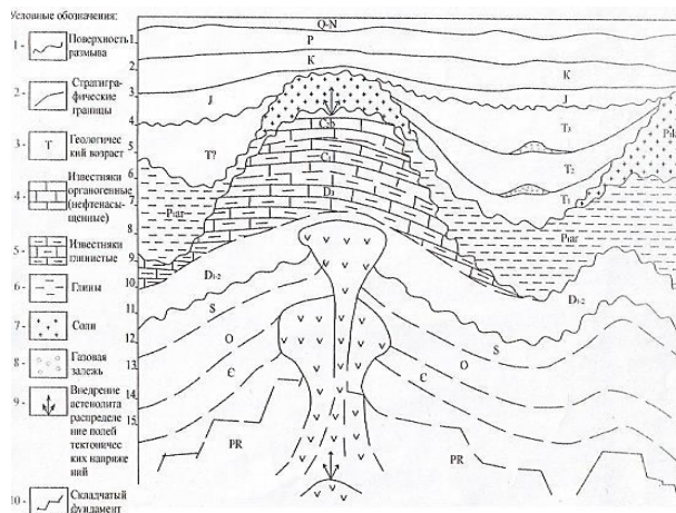
Рис. 2 Геолого-тектоническая модель Нурин-Хагской перспективной площади на нефть и газ
