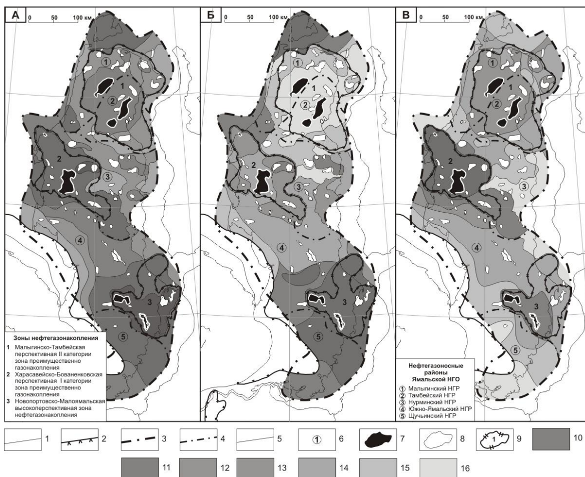
Рис. Карты перспектив нефтегазонаосности (А), нефтеносности (Б) и газоносности (В) батского регионального резервуара Ямальской НГО
