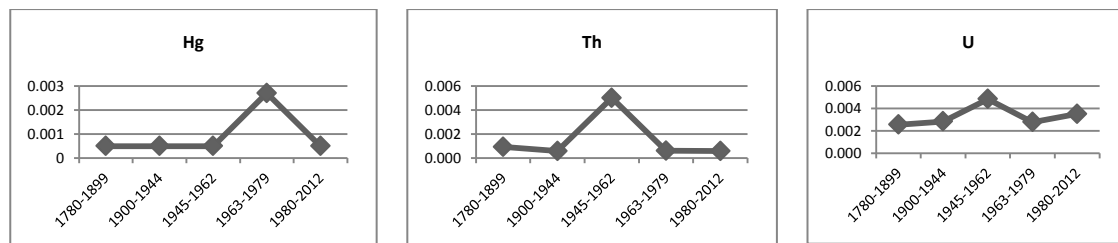
Рис. 3 Диаграммы содержаний химических элементов Hg, Th, U (мг/кг) на интервале с 1780 по 2012 годы
