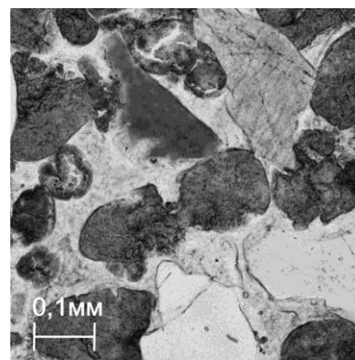
Рис. 3. Песчаник кварцево-глауконитовый на кремнистом цементе
