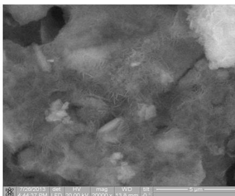
Рис. Электронная микрофотография торфомагнезиальных композиций, твердевших в воде
