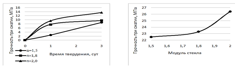
Рис. 1. Зависимость прочности образцов: а) от продолжительности твердения б) от модуля стекла после обжига при температуре 1000 °С
