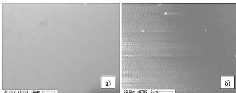
Рис.3. Поверхность стеклокристаллического покрытия с добавкой в исходную шихту 1,5 мас.% \text{CeO}_2 : а) материал не подвергнутый химическому травлению (Т спек.=1250 °С); б) материал, подвергнутый химическому травлению (Т спек.=1250 °С)
