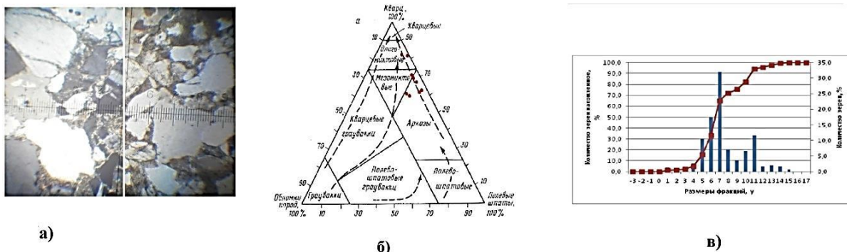
Рис. 2. Пример фотографии шлифа, результатов минерально-петрографического и гранулометрического анализа: а) фото шлифа при увеличении \times 25 (слева // николи, справа +); б) диаграмма В.Н. Шванова; в) гистограмма распределения зерен по фракциям и кумулятивная кривая для образца 3 (см. рис. 1)
