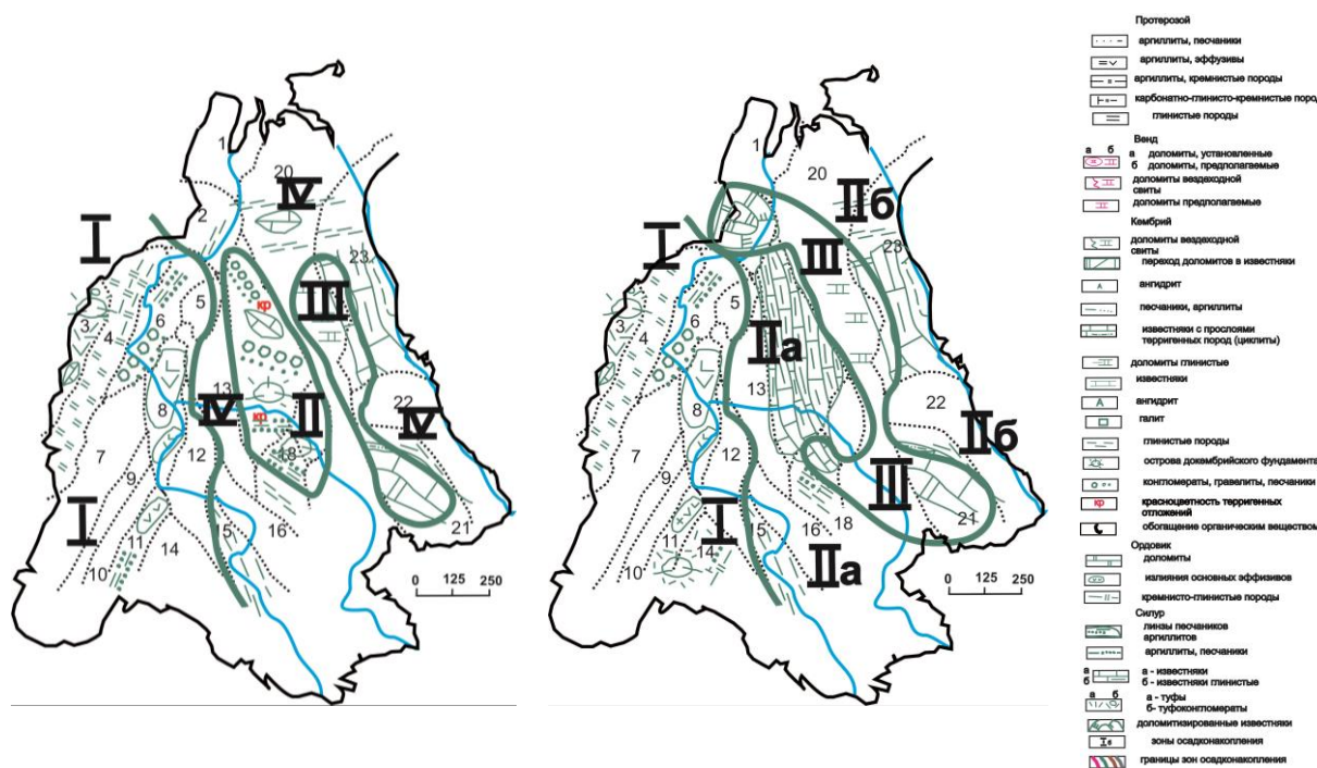
Рис. Палеогеографическая карта распространения нижне- и средне-верхнеордовикских отложений на территории Западно-Сибирской геосинеклызы:
