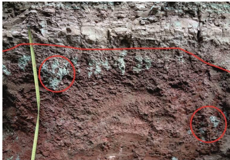
Рис.2 Почвенный горизонт (в слое красной глины видны пятна оглеения по корневым пустотам)
