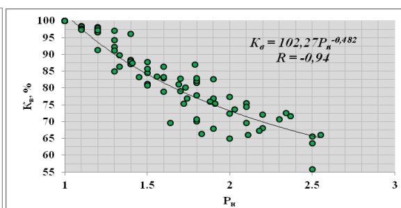
Рис. 2. Петроэлектрическая модель насыщенности для терригенных пород разреза
