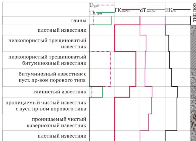
Рисунок 1. Схематические диаграммы доступного комплекса ГИС в породах различных типов
