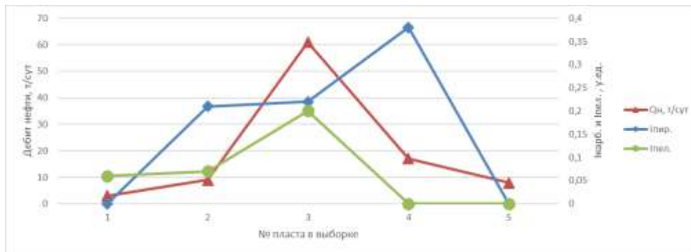
Рис. Сравнение дебита нефти ( Q_n ), пиритизации ( I_{пир.} ) и пелитизации ( I_{пел.} ) пластов Ю 1
