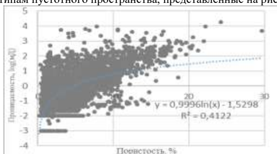
Рис. 1. Зависимость проницаемости от пористости по всем образцам керн
