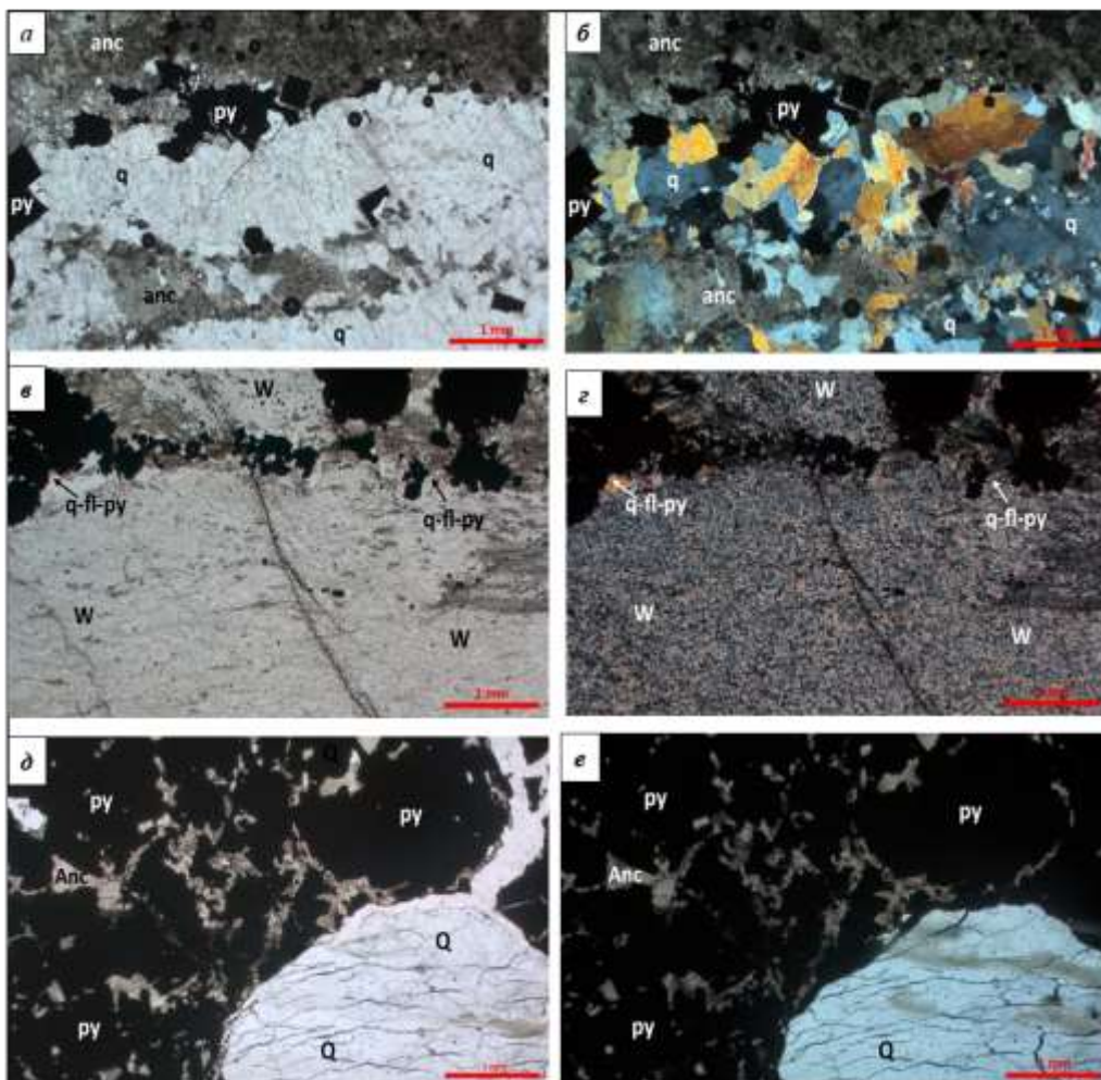
Рис. Типы рудной минерализации в метасоматитах: вкрапленный (а, б), прожилково-вкрапленный (в, г), густо-вкрапленный (д, е). Условные обозначения: а, в, д – съемка при одном никеле, б – в скрещенных. Anc – анкерит, q – мутный кварц, py – пирит, Q – молочно-белый кварц, W – тонкозернистый кварц во вторичном кварците, q-fl-py – кварц-флюорит-пиритовый агрегат
