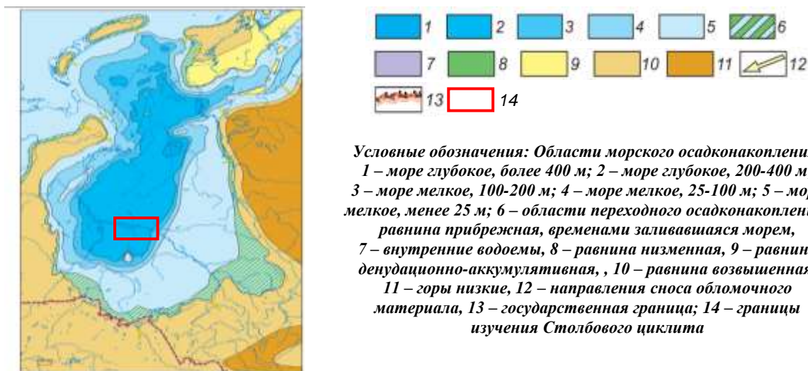
Рис. 2. Палеогеографическая схема Западно-Сибирской провинции на конец берриаса-начало валанжина [3]
