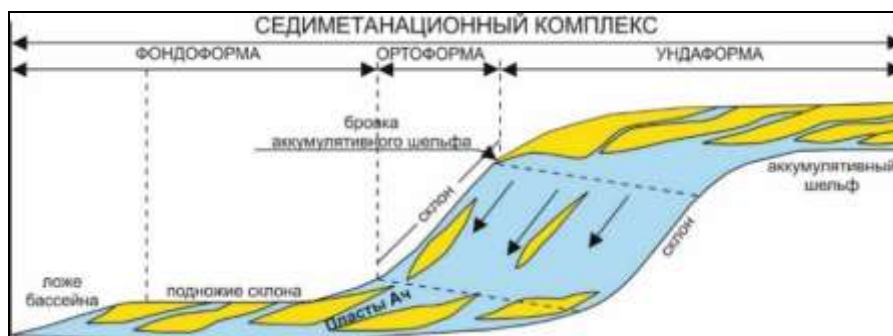
Рис. 1. Схема формирования клиноформного комплекса пород
