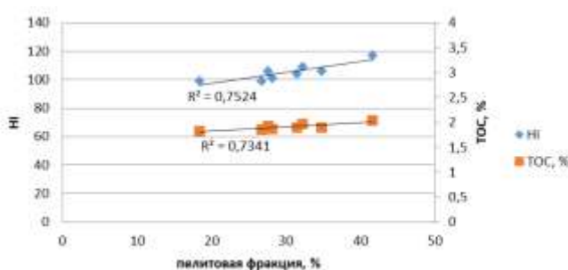
Рис. 2. График зависимости между параметрами TOC, HI и содержанием пелитовой фракции
